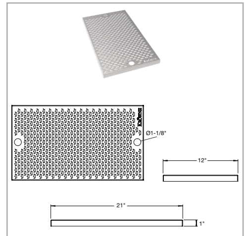
MW-DB12 - MoveWell Drainboard, 12"W
